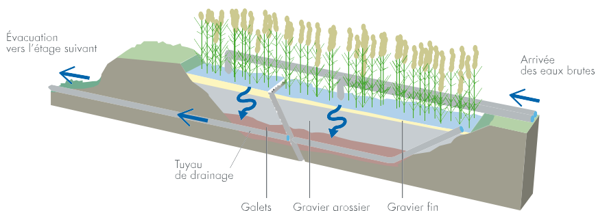
Schéma filtre planté - Source CEMAGREF
